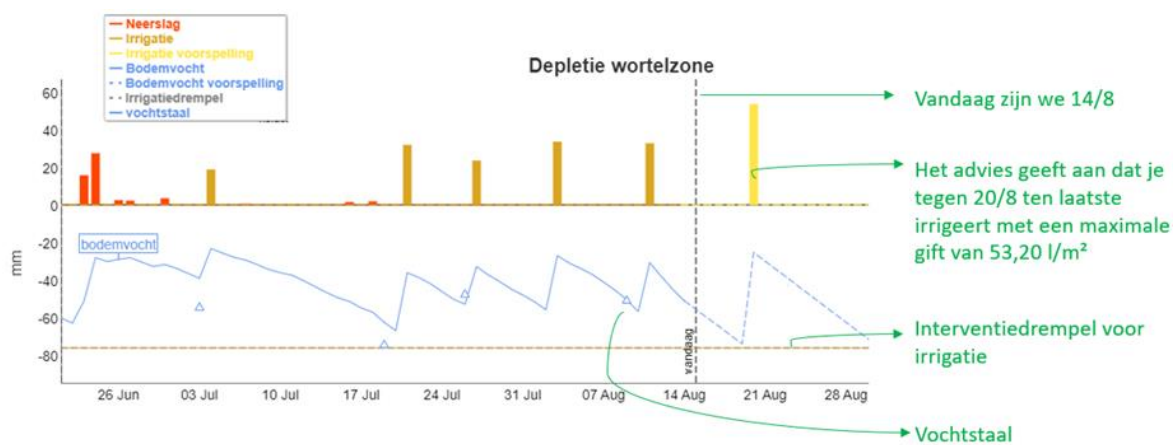
Figuur 6. Resultaat van het irrigatieadviesmodel voor het aspergeperceel te Kinrooi. De depletie in de wortelzone (blauwe lijn) wordt berekend door het model. Dit vormt de basis om een irrigatieadvies uit te sturen.
