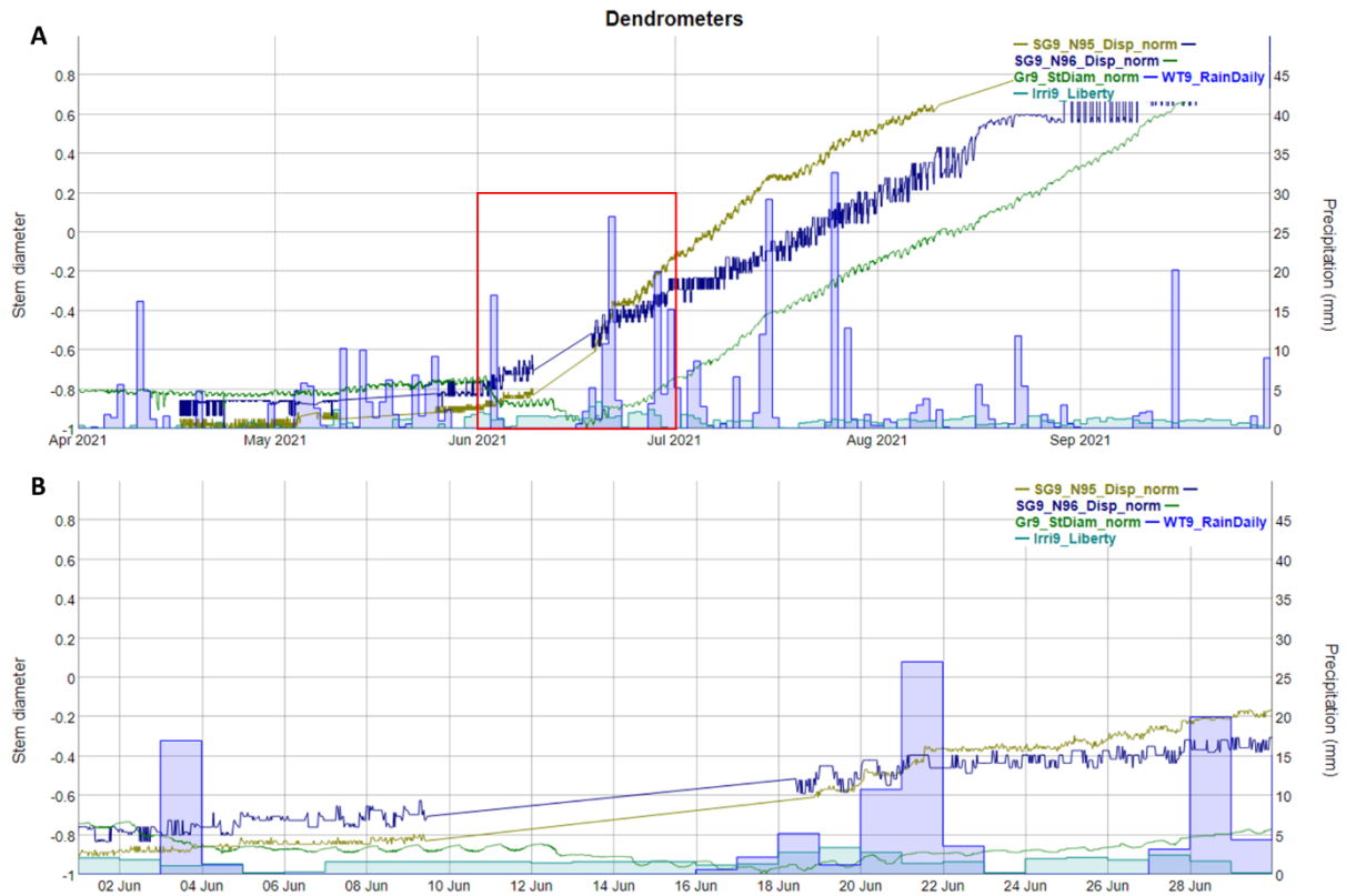
Figuur B. 47. Resultaten voor de stamdiameter (herschaald tussen -1 en 1) gemeten door sensornodes 95 (geel) en 96 (blauw) en door de sensor van 2Grow (groen) op het blauwe bessenperceel te America in 2021. Neerslag en irrigatie worden weergegeven door respectievelijk donker- en lichtblauwe balken (boven). B. Detail voor de periode juni 2021.
