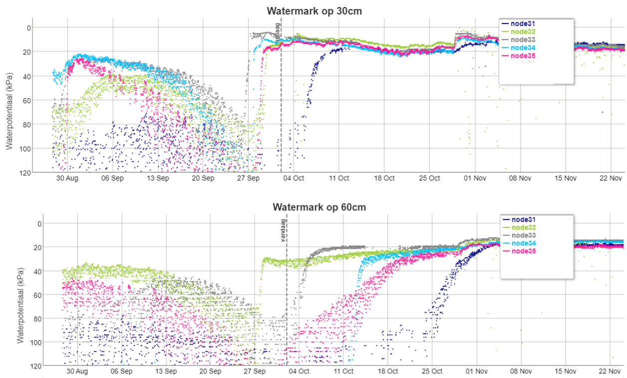
Figuur B. 13. Resultaten van de Watermarksensoren op 30 cm (boven) en 60 cm (onder) voor het aspergeperceel te Booischot in 2020. De verschillende kleuren stellen de vijf sensornodes voor.
