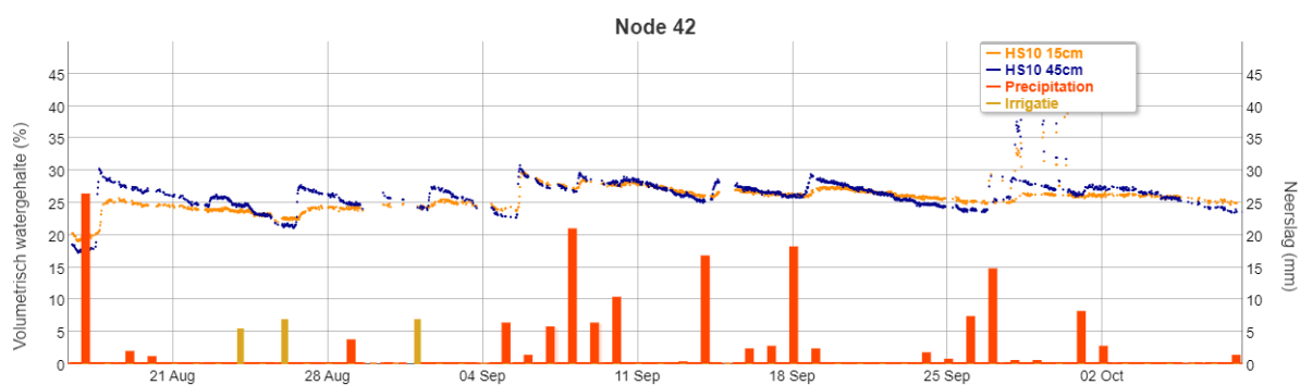
Figuur B. 21. Resultaten van de 10HS-sensoren voor node 42 op het prunusperceel te Venlo in 2022. De twee sensoren werden omgewisseld: blauw = 15 cm diepte, oranje = 45 cm diepte.
