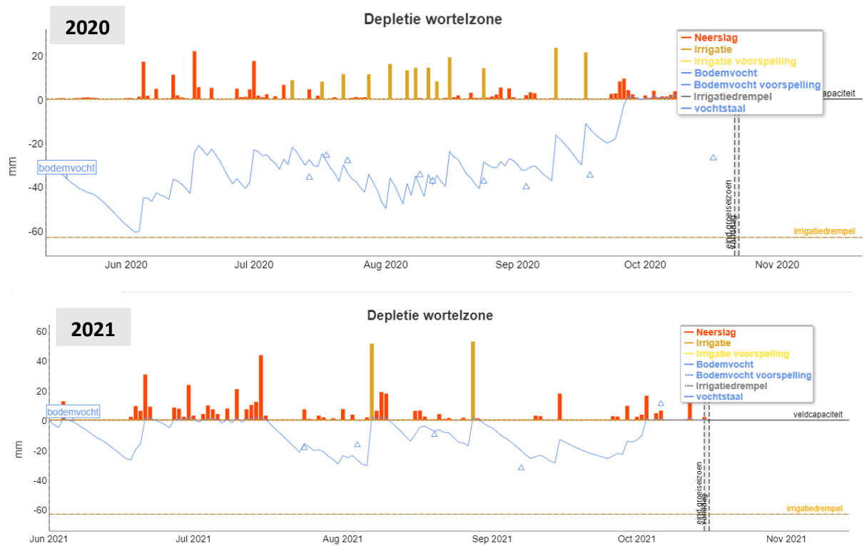
Figuur B. 5. Simulatie van het bodemvocht in de wortelzone (blauw) vergeleken met bodemstalen (driehoekjes) voor het aspergeperceel te Peer in 2020 en 2021.
