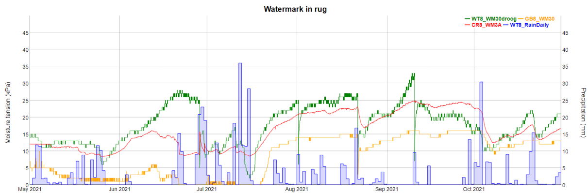
Figuur B. 36. Resultaten van de Watermarksensoren aangesloten op het systeem van Wolky Tolkly (groen), Geobas (oranje) en Crudeon (rood) voor het blauwe bessenperceel te Oudsbergen in 2022. De blauwe balken geven de neerslag weer.
