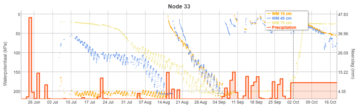
Figuur B. 14. Resultaten van de Watermarksensoren voor de verschillende bodemlagen op eenzelfde node voor het aspergeperceel te Booischot in 2022.
