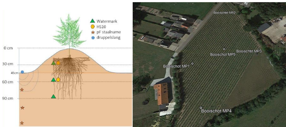
Figuur B. 12. Plaatsing van de sensoren op het aspergeperceel te Booischot in de diepte (links) en verspreid over het perceel (rechts).
