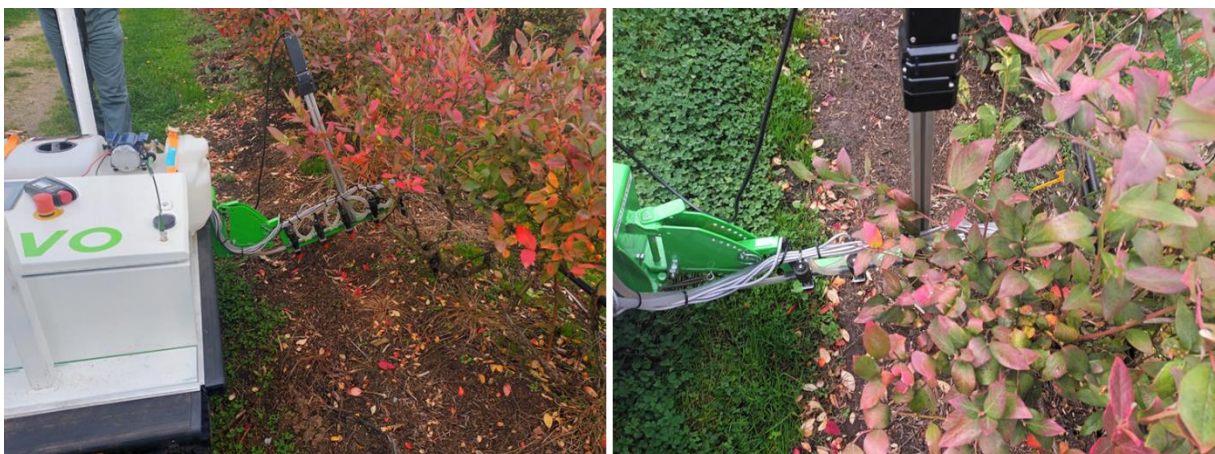
Figuur 7. Test met de Treebot op het blauwe bessenperceel te Oudsbergen (B) op 24/10/2022. De onderste takken van de struiken komen tussen de spuitboom en de camera waardoor de spuitdoppen onnodig aangeschakeld worden.
