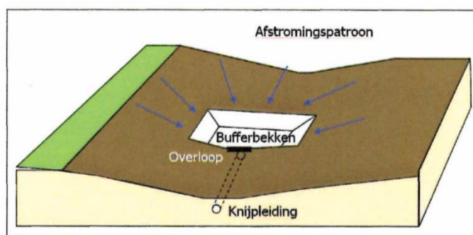
Figuur 7. – Principe van een bufferbekken (LNE, 2010).
